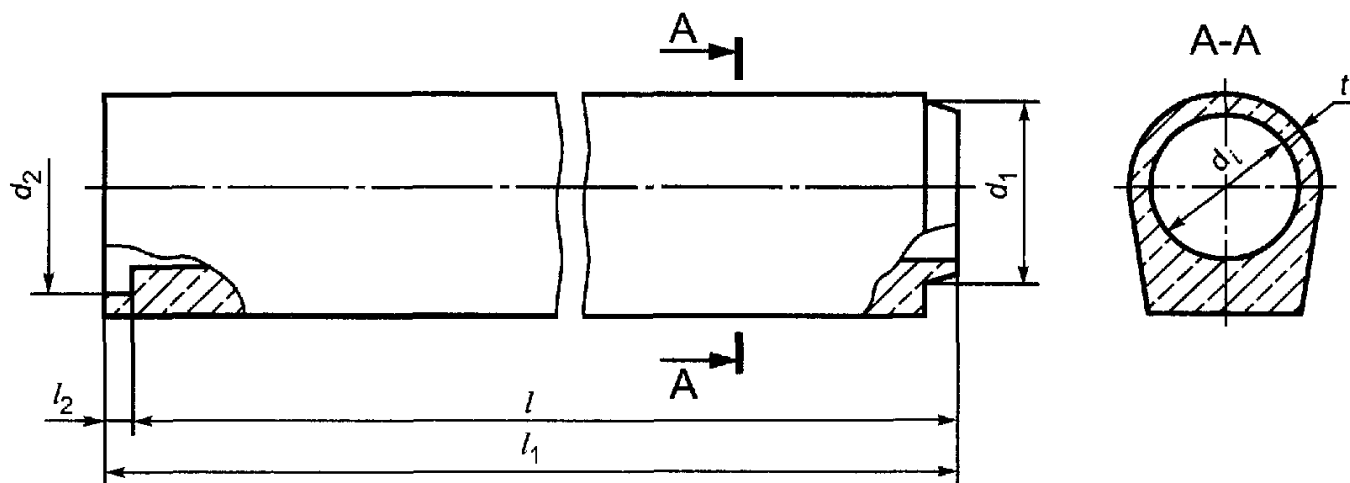
Рисунок А.6 — Общий вид труб типа ТФП
