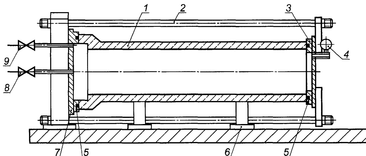
1 — труба; 2 — тяжи; 3 — подвижная заглушка; 4 — манометр; 5 — уплотнительные прокладки; 6 — опора; 7 — неподвижная заглушка; 8 — вентиль подачи воды; 9 — вентиль выпуска воздуха
