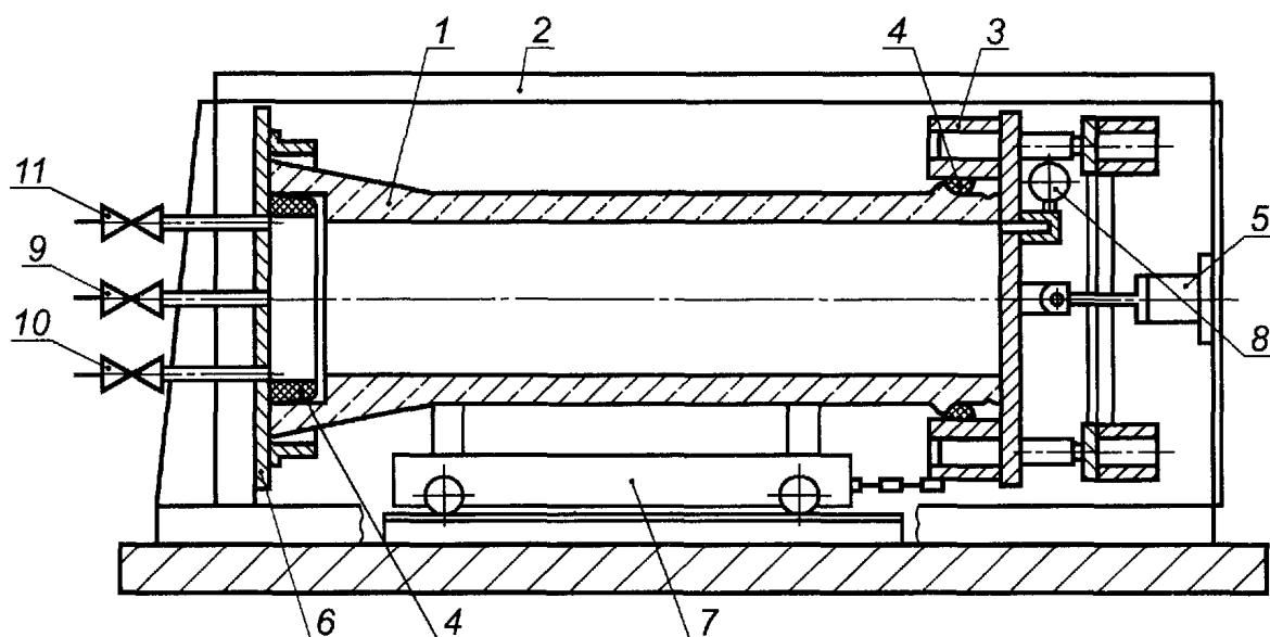
1 — труба; 2 — рама гидростенда; 3 — подвижная заглушка; 4 — уплотнительные кольца; 5 — гидроцилиндр; 6 — неподвижная заглушка; 7 — тележка; 8 — манометр; 9 — вентиль подачи воды; 10 — вентиль слива воды; 11 — воздушный вентиль
