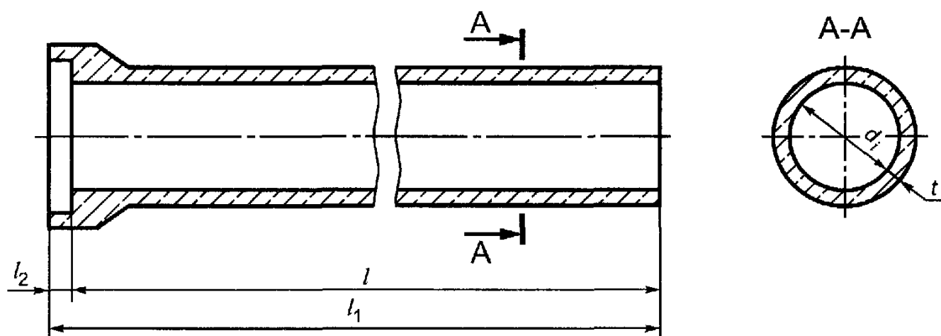
Рисунок А.1 — Общий вид труб типа Т
