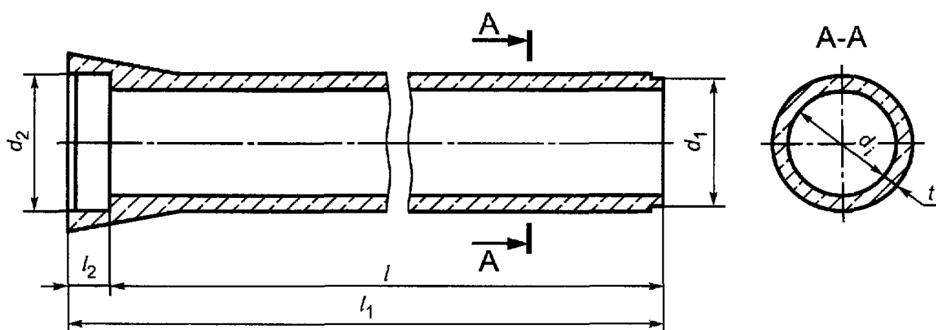
Рисунок А.2— Общий вид труб типов ТБ и ТС
