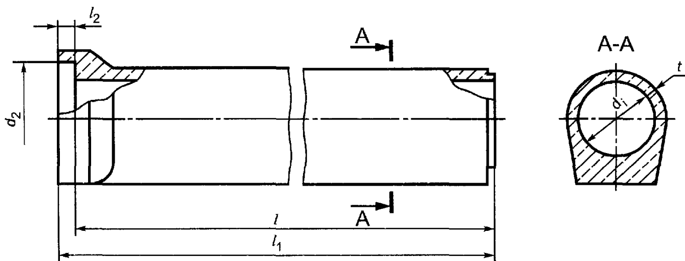
Рисунок А.4 — Общий вид труб типа ТП
