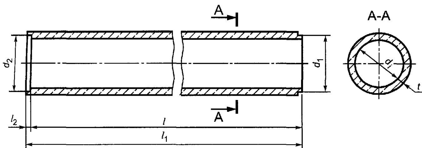
Рисунок А.3— Общий вид труб типа ТФ
